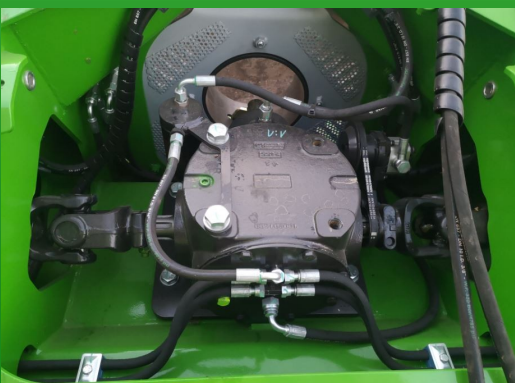
Système de lubrification avec pompe et filtre
